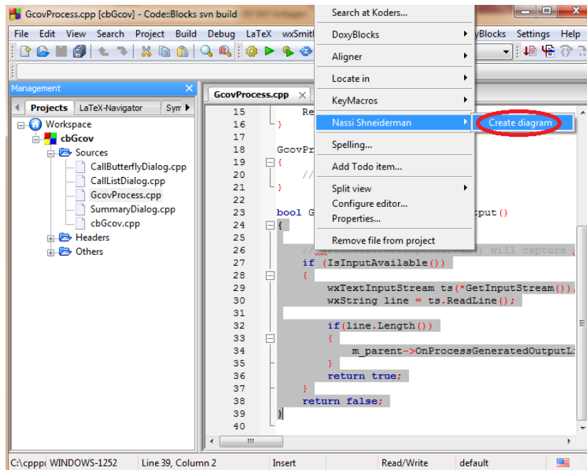
Figure 2.16: NassiShneiderman Création
